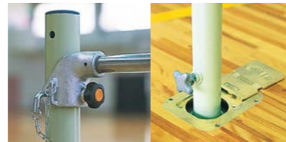
バー受部
