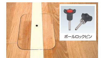
VT-6658 バレー・テニスポスト用床金具<弾性シート貼>
